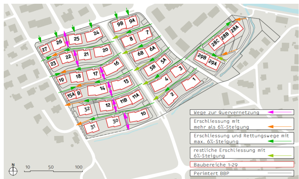
Situation Erschliessungs- und Rettungskorridore (Quelle: Planungsbericht Bebauungsplan Zimel Art. 47 RPV vom 16.12.2015)
