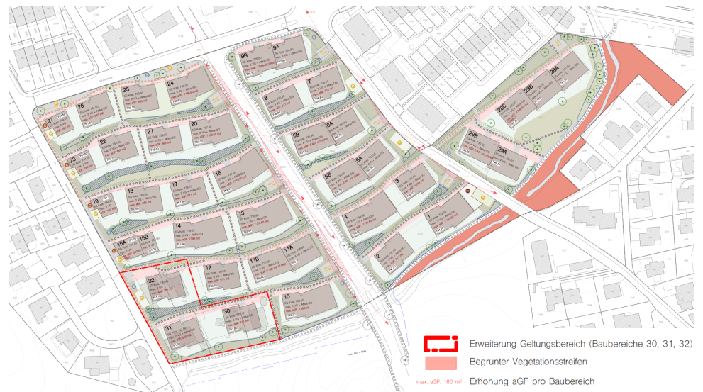
Änderungsplan ordentlicher Bebauungsplan Zimel (Quelle: KEEAS AG)
