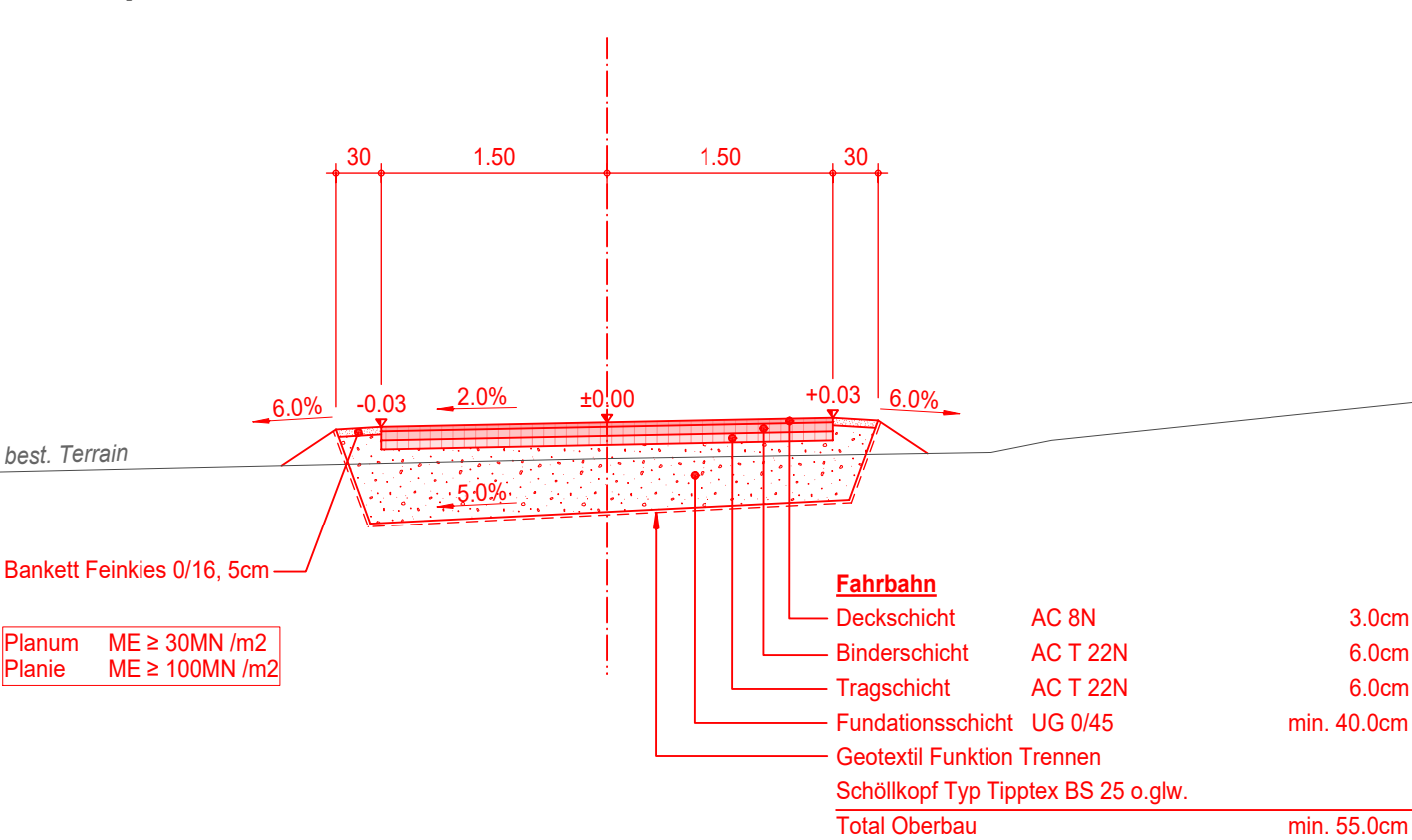
Normalprofil Strasse, 1:50
