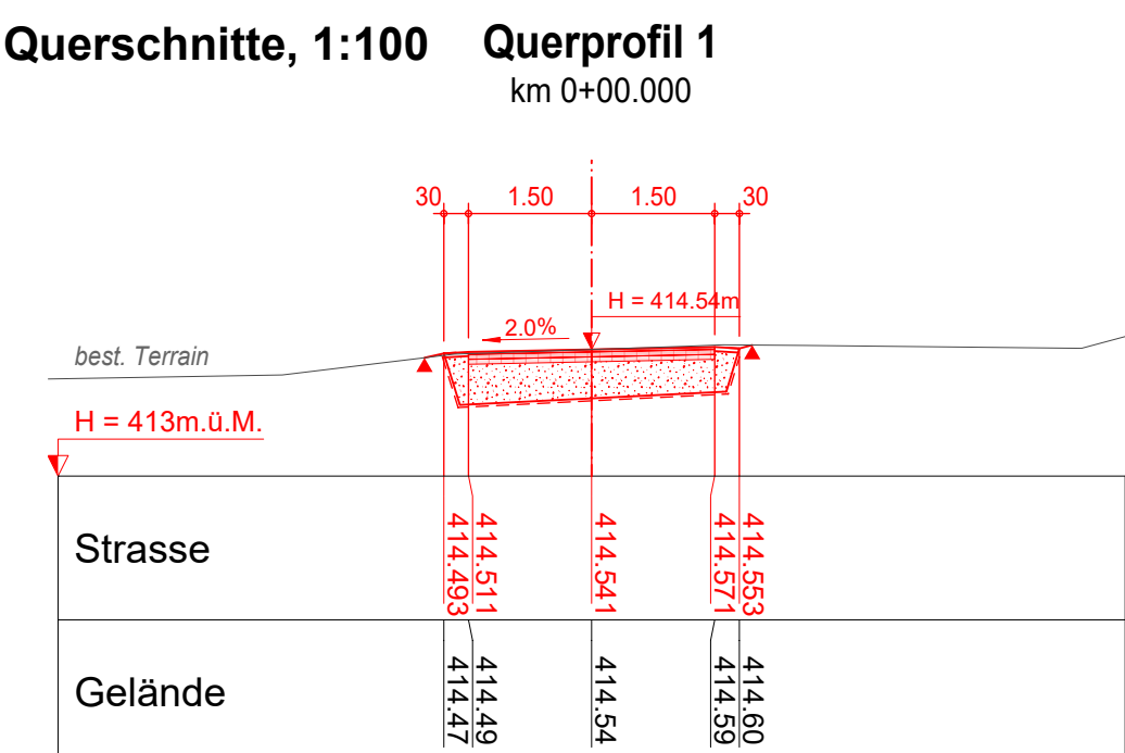
Quersprofil 4
