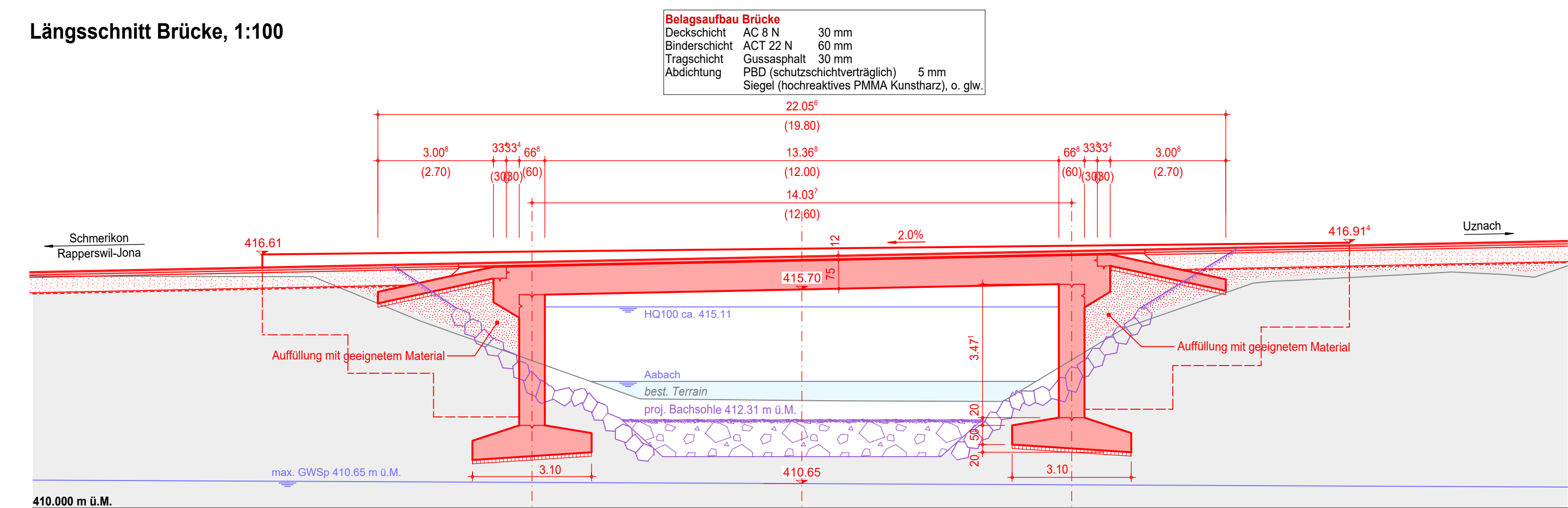
Längsschnitt Brücke, 1:100
