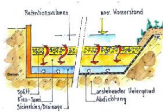
Abbildung 6: technische begrünte Retentionen (SABA)
