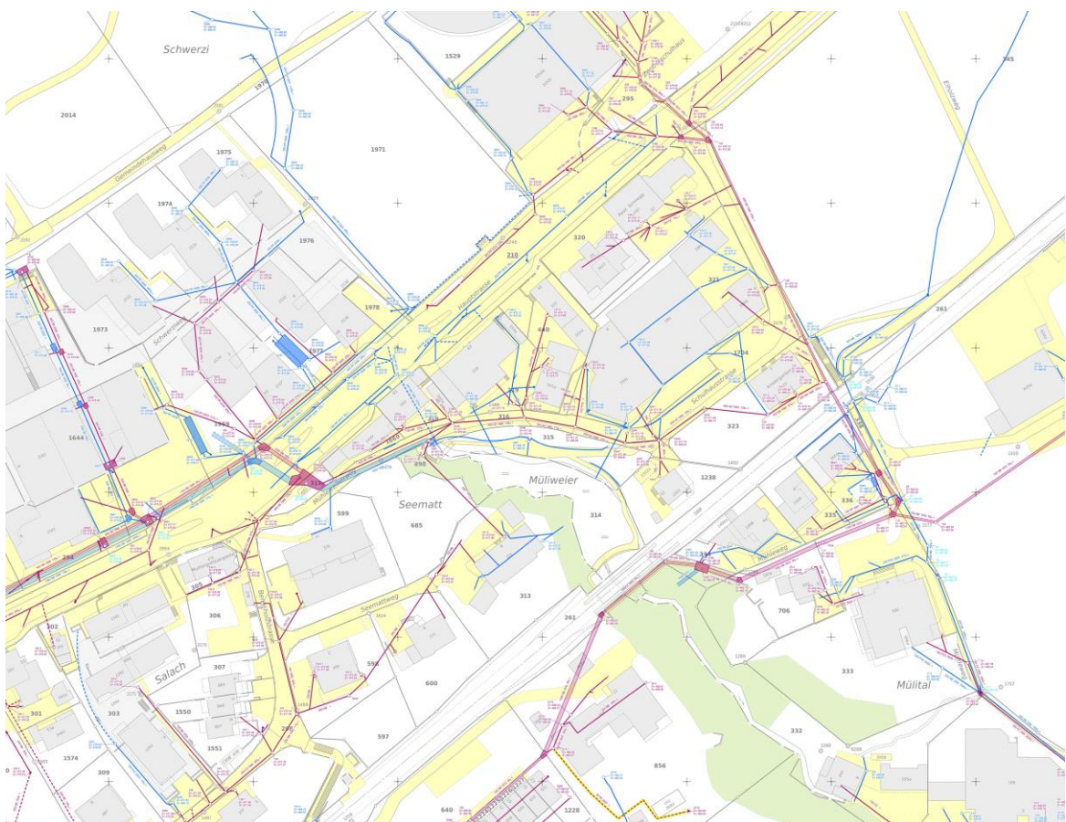
Abbildung 2: Ausschnitt bestehender Abwasserkataster
