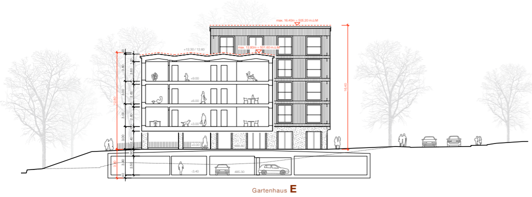
Gartenhaus E
