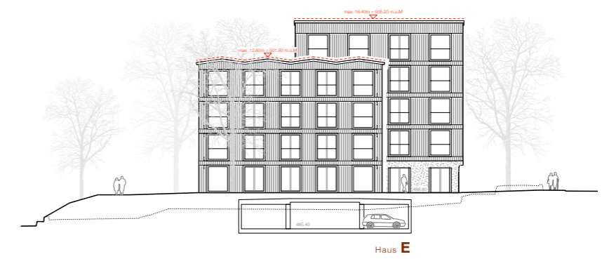
ANSICHT WEST HAUS E
