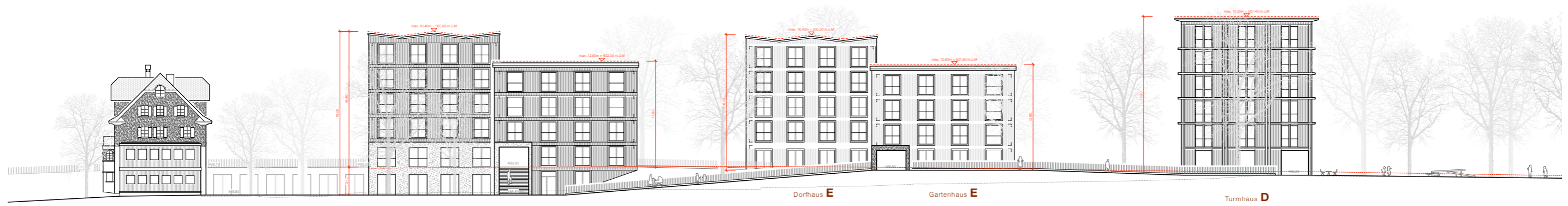
ANSICHT NORD (TEIL LINKS)
