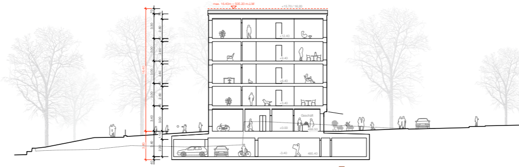
Dorfhaus E
