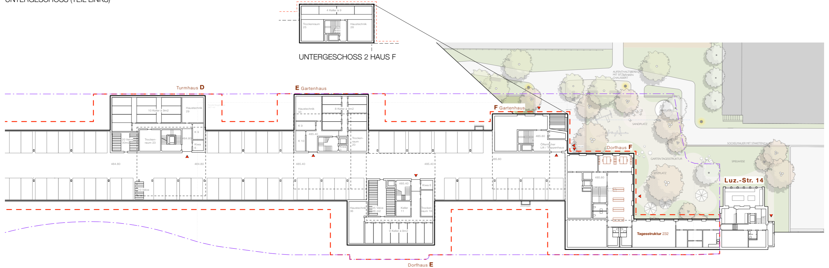
UNTERGESCHOSS OST (TEIL RECHTS)
