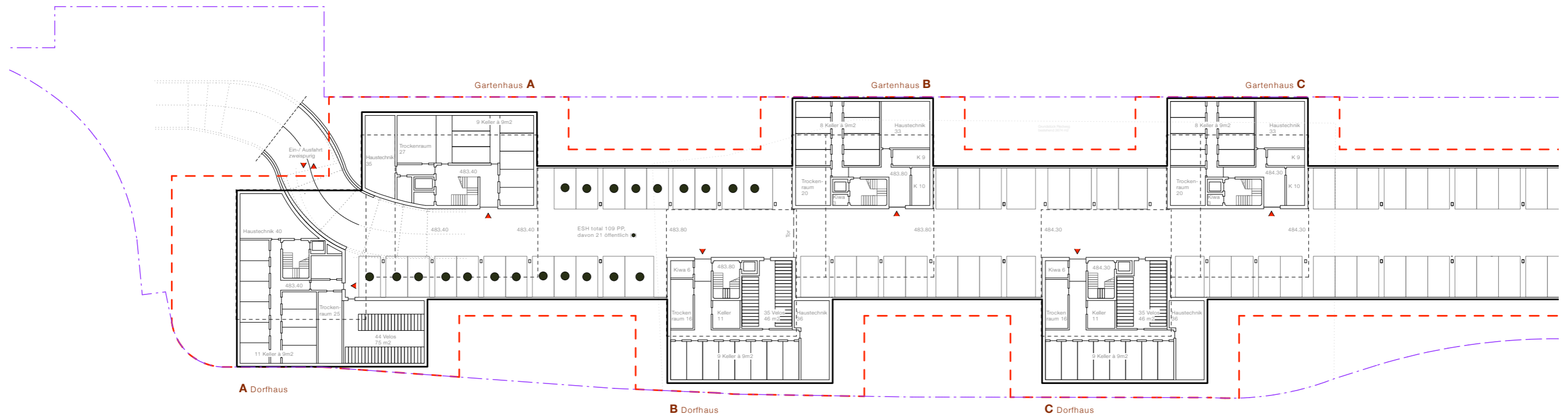
UNTERGESCHOSS (TEIL LINKS)
